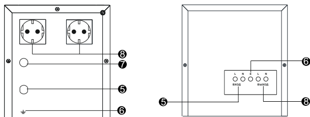
Задняя панель
