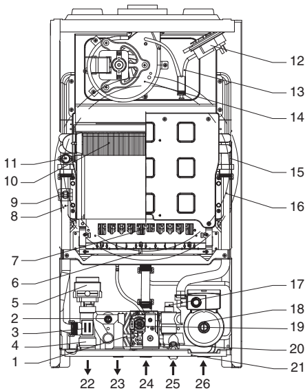
Внутренняя структура котла
