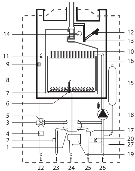
Принципиальная схема
